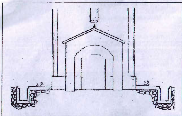
Шема хидроизолације около манастирске цркве
