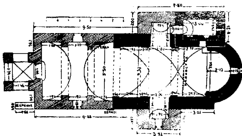
Основа цркве
